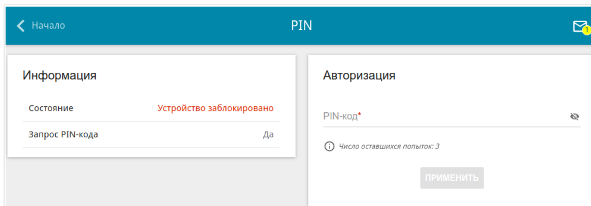
Рисунок 126. Ввод PIN-кода.
