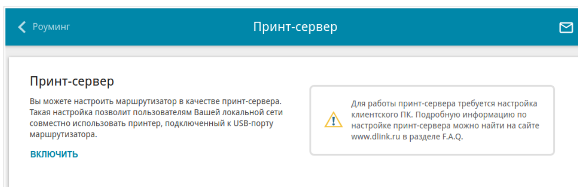
Рисунок 111. Страница Принт-сервер .
