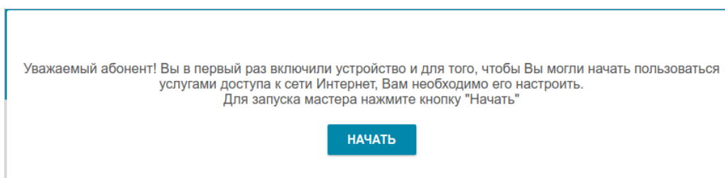
Рисунок 20. Запуск Мастера.
