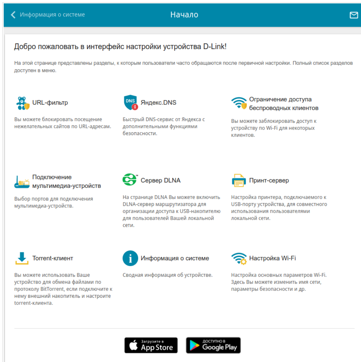
Рисунок 16. Страница Начало .
