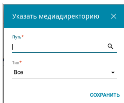
Рисунок 120. Добавление медиадиректории.
